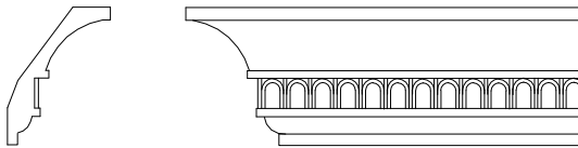
CCR19 8"X 6"
