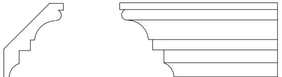
CCR27 9"X 7"
