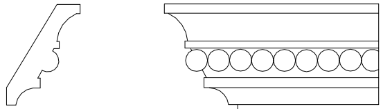
CCR25 9"X 6.5"
