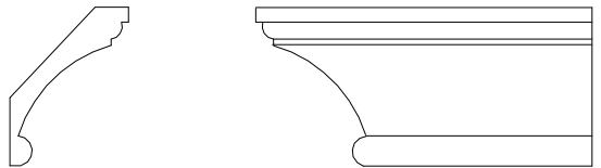
CCR26 9"X 7"
